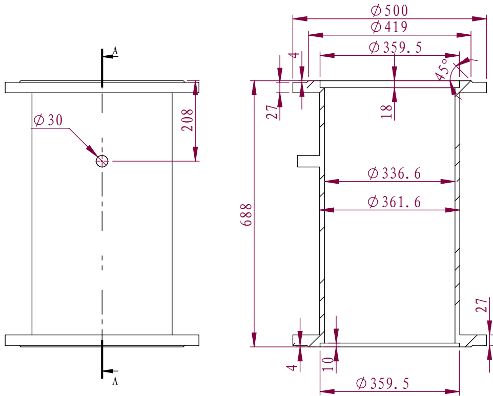
剖面 A-A 比例 1 : 10
